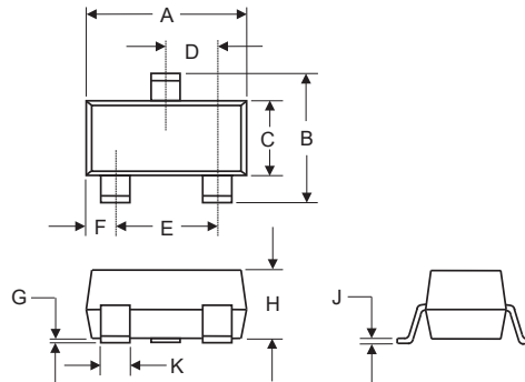
SOT-23-3L
